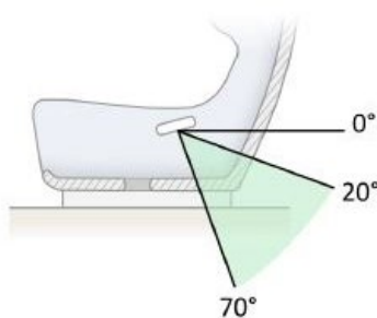
Dessin / Drawing 253-61-b
